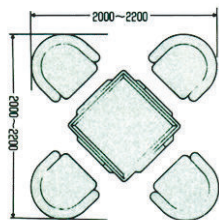
配置寸法図
